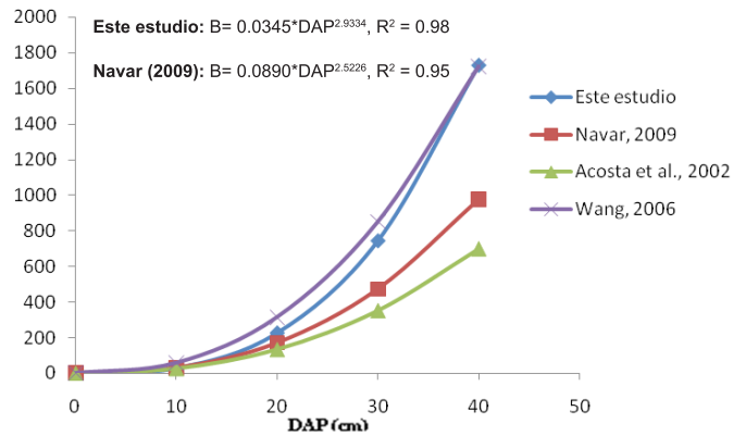
FIGURA 2. Modelos para la estimación de biomasa en función del diámetro a la altura del pecho para el género Quercus
