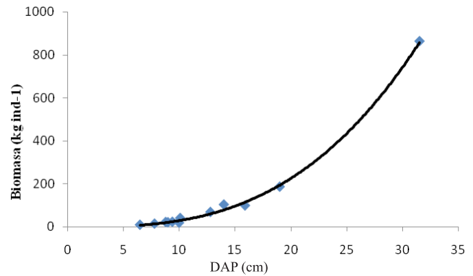
FIGURA 1. Dispersión de los datos y línea de tendencia de los valores reales de Biomasa aérea para Quercus magnoliaefolia Née
